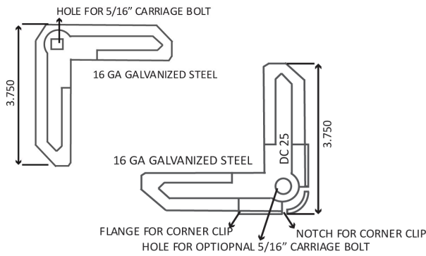
D25 CORNER W/CLIP
