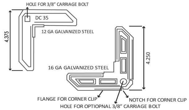
D35 CORNER W/CLIP
