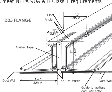
D25 CORNER W/NUT & BOLT
