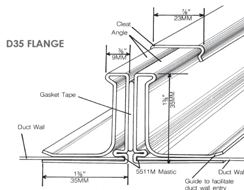
D35 CORNER
